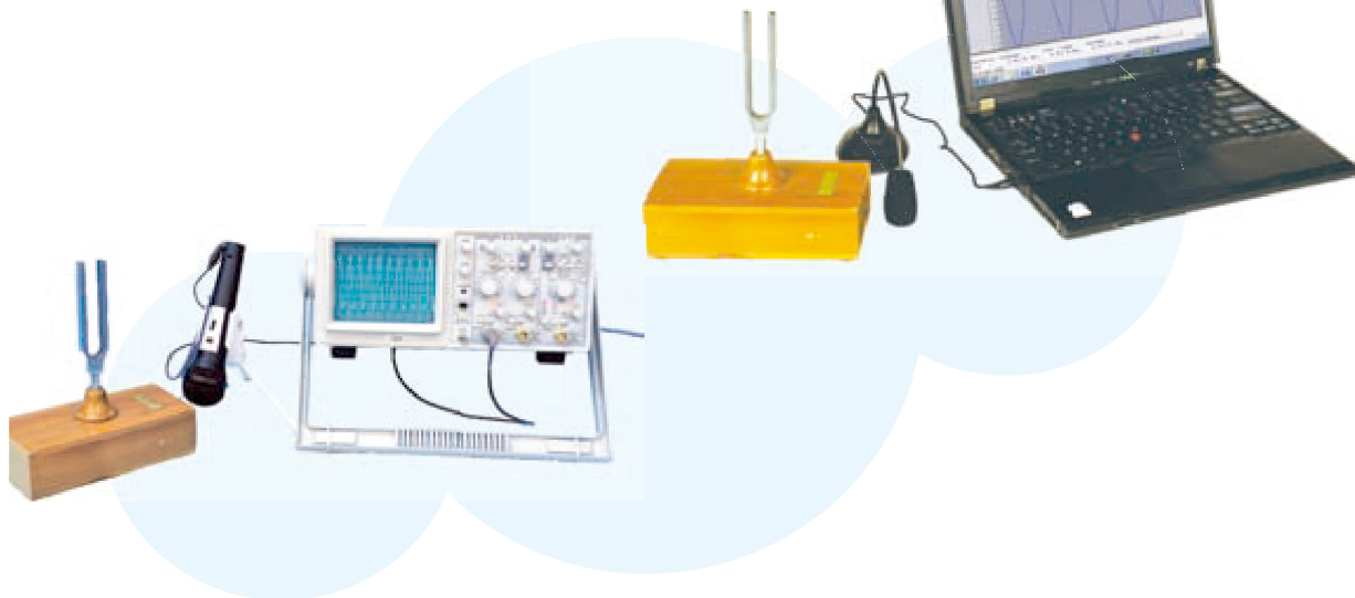
图 2.2-2 声音的波形
