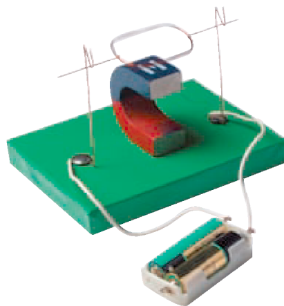
图10 通电的线圈放在磁场中会转起来，为什么？
