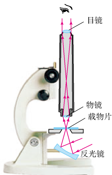
图5.5-1 显微镜的结构
