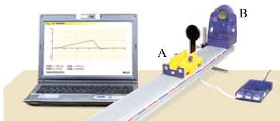
图1.4-2 实验装置
