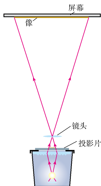
图5.2-3 投影仪成像原理
