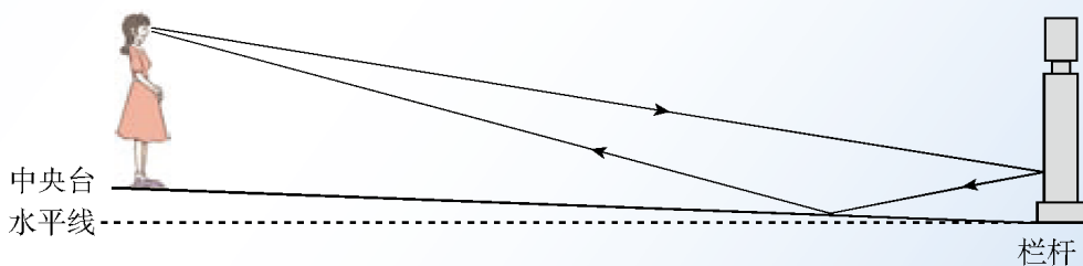
图2.3-9 圜丘反射声的示意图
