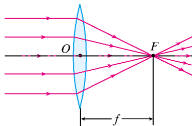
图5.1-7 凸透镜的焦点和焦距
