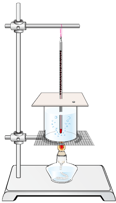
图 3.3-2 观察水沸腾的装置
