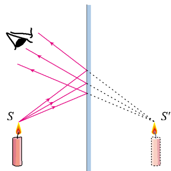
图4.3-3 平面镜中的像是虚像
