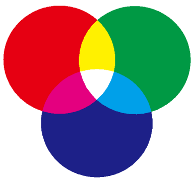
图4.5-3 色光的三原色
