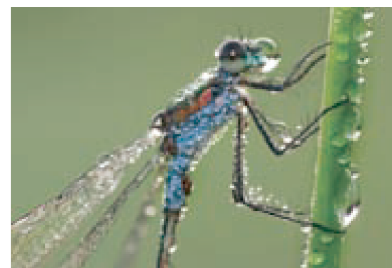
图 3.3-6 昆虫和植物上的露珠
