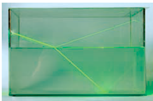
图4.4-1 光射入水中时的折射现象
