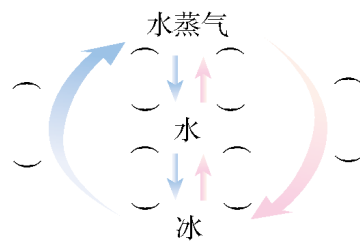
图 3.4-2 水的三态联系
