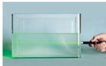
图4.1-2 光在水中的传播
