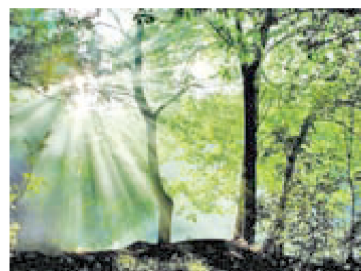
图4.1-1 光在空气中沿直线传播
