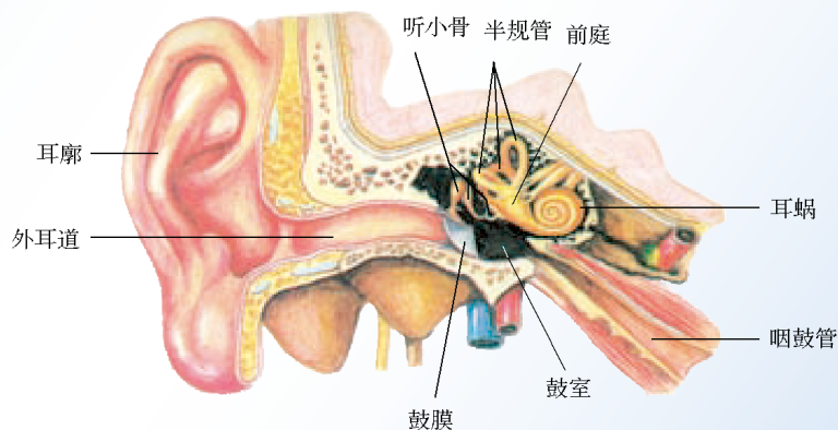
图2.1-8 人耳构造
