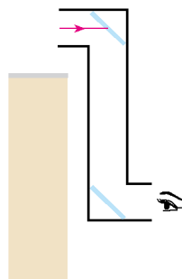
图4.3-12 潜望镜
