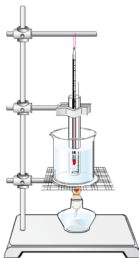
图3.2-1 观察熔化现象的实验装置
