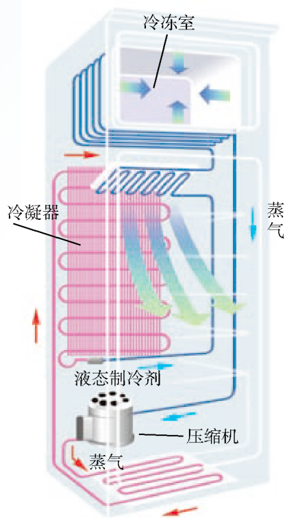
图3.3-8 电冰箱原理图
