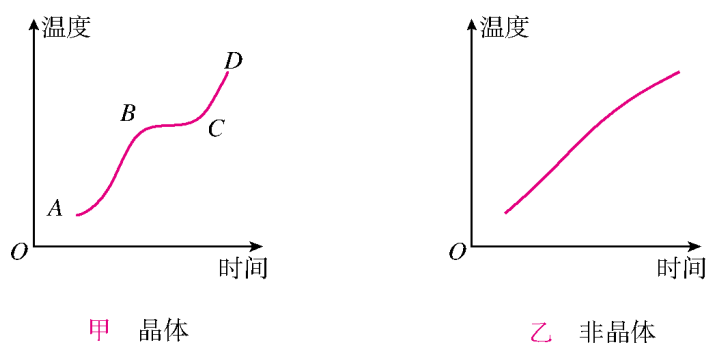
图 3.2-4 物质熔化时的温度变化曲线
