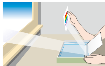
图4.5-2 光的色散实验
