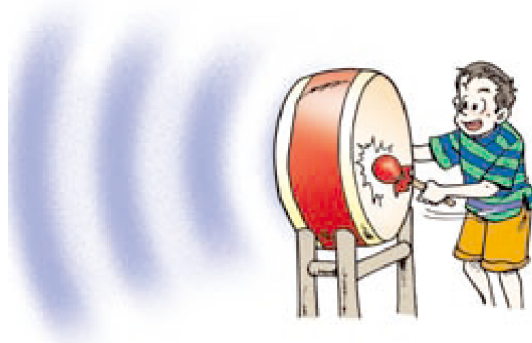
图2.1-6 空气疏密部分的传播形成声波
