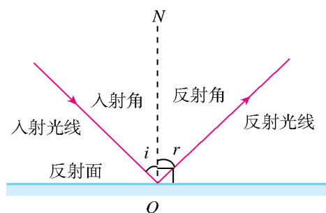
图4.2-4 光的反射
