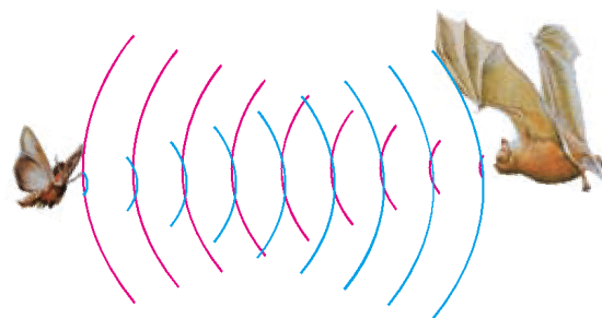
图2.3-2 蝙蝠靠超声波发现昆虫
