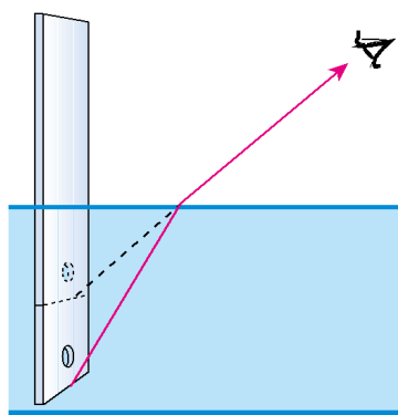
图4.4-3 池水变“浅”了
